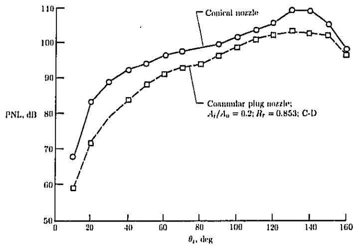
(d) PNL directivity characteristics.
